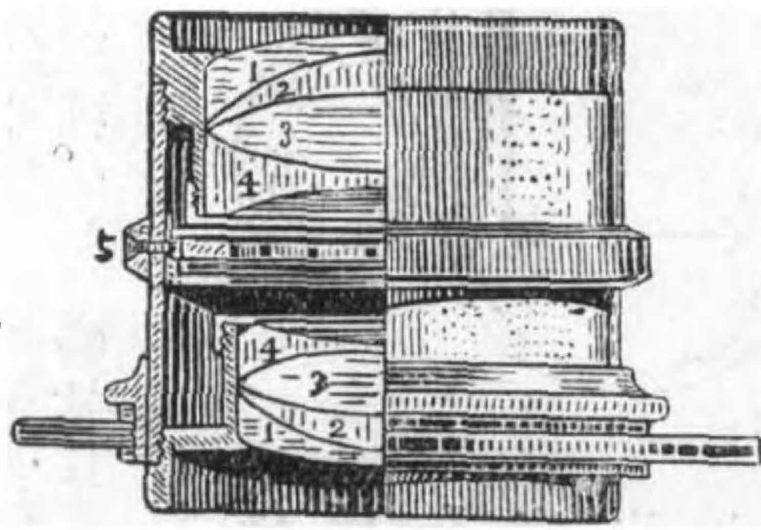
示撥羅泰式鏡 頭之剖面 1 為火石玻璃 2 及 4 為折光 較弱之冕號 玻璃 3 為折光較強 之冕號玻璃 5 隔簾式之鎖 光圈
