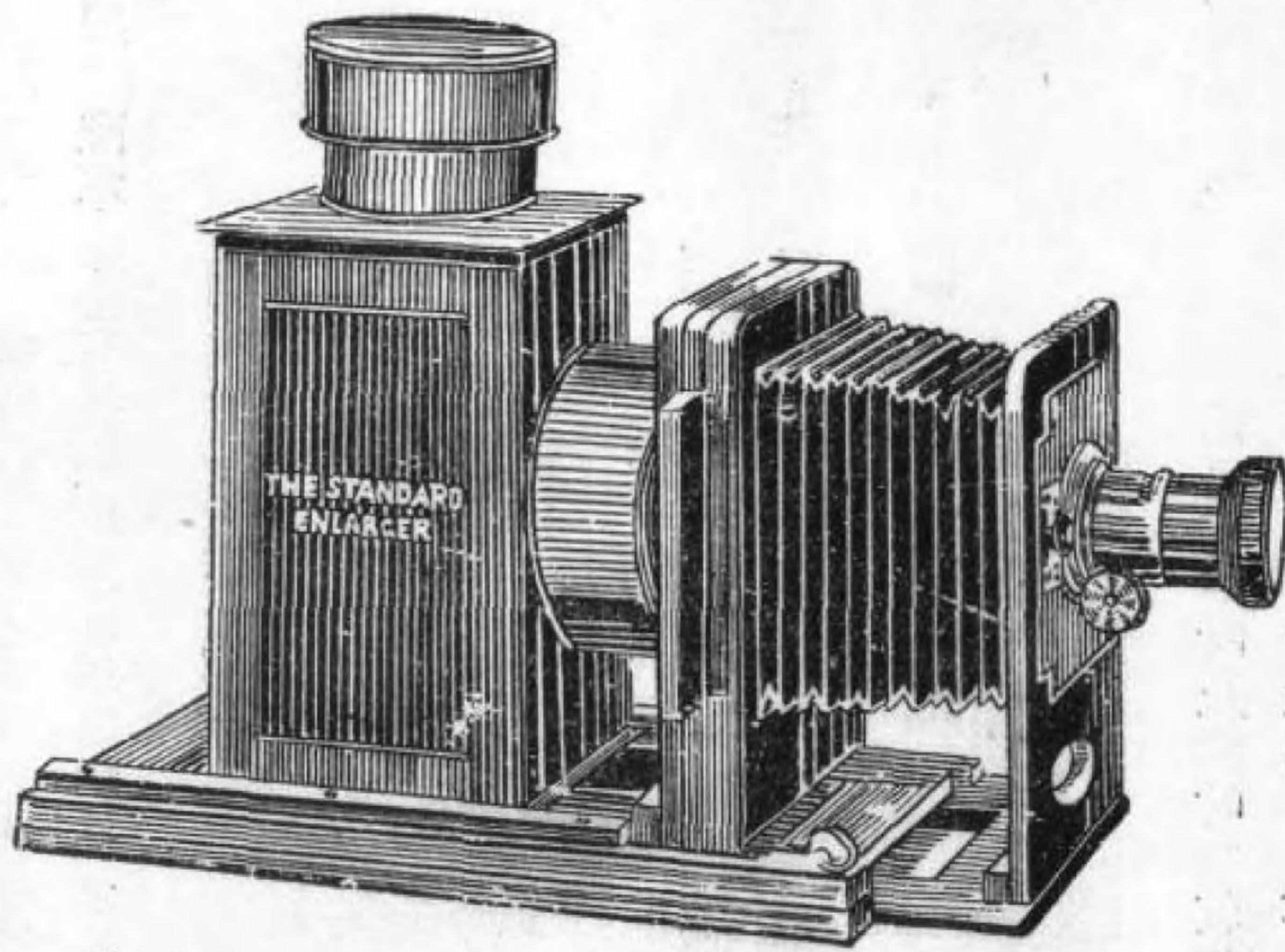
放大燈前有鏡頭及鑿腔後有線之燈
