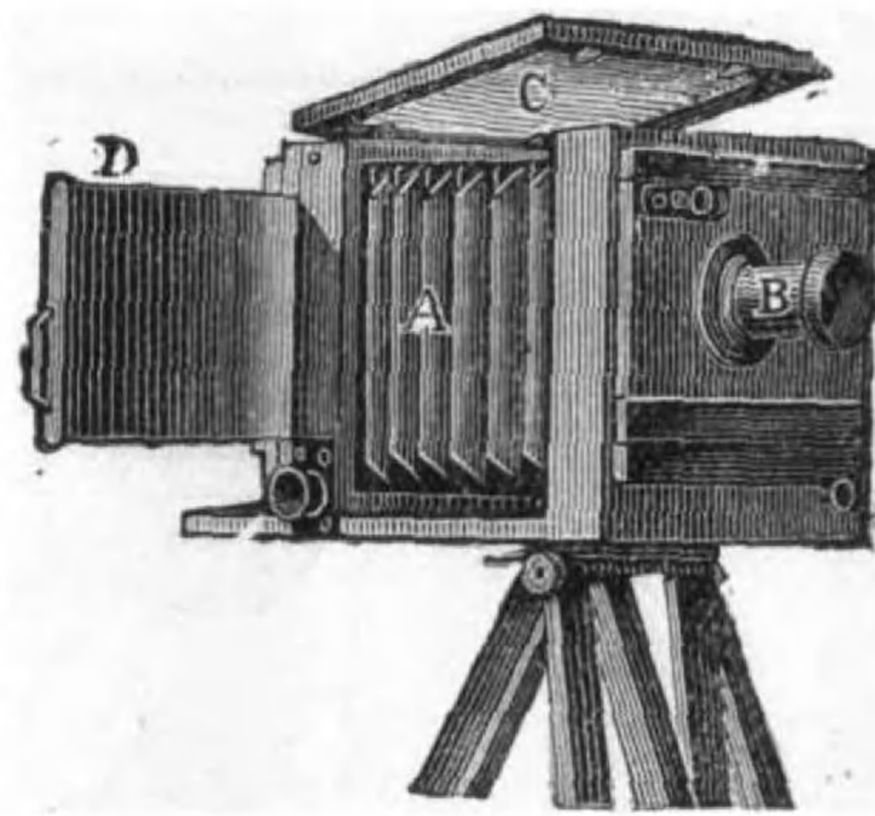
示攝影時裝置器具式 A 為暗箱之裝腔可進退以配光距 B 為鏡頭前方有蓋 C 為承影玻片物影即落於此以察光距之配準與否是圖承影玻片翻在上面因暗匣已插入暗箱 D 為暗匣之門已向外抽出而匣中乾片正對鏡面
