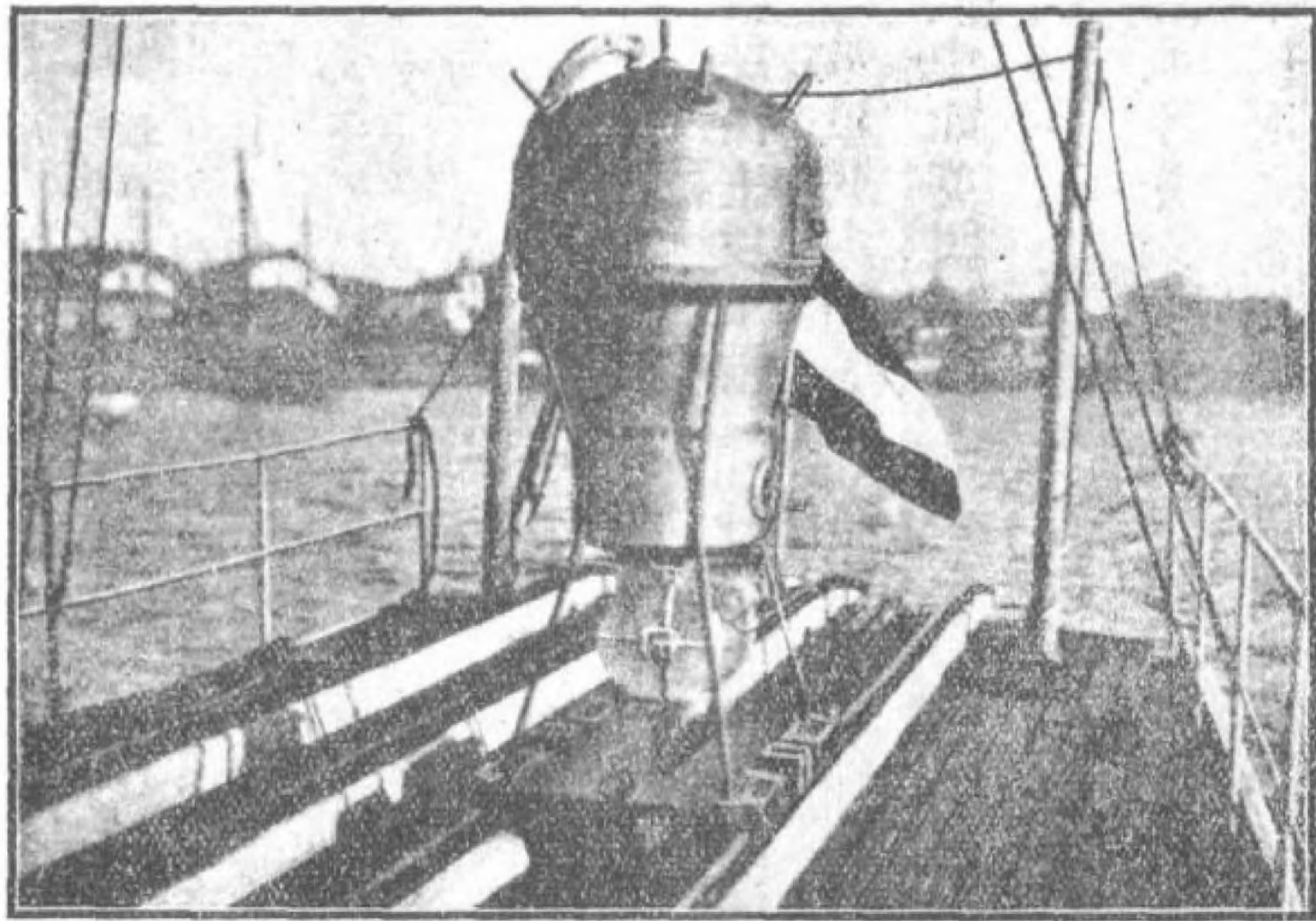
圖之上艦雷水埋在雷水式 Trotyl 國德
