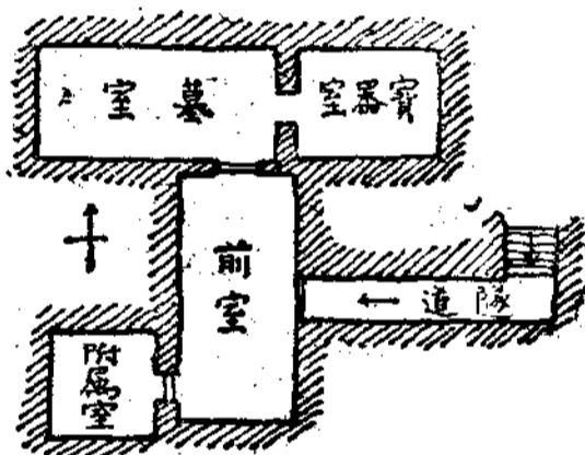
都丹喀門王之陵之平面構造
