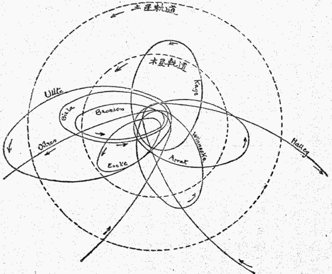
圖五 (彗星的軌道)
