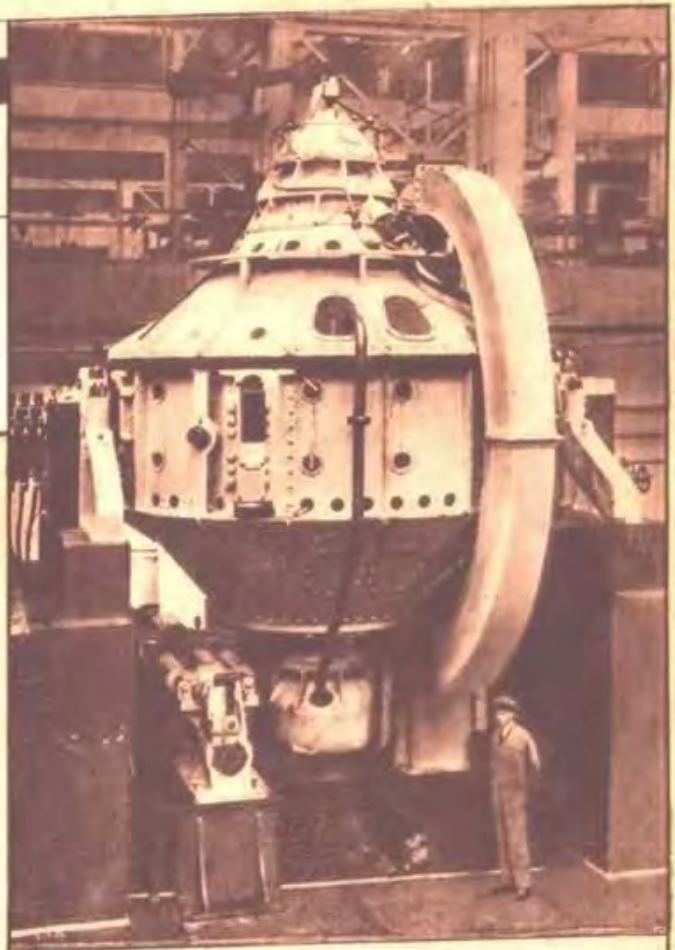
上圖即為法國商輪「諾曼第」號之正視。為求旅客之舒適，最近意大利打造一艘商船，名為 Conte di Savoia。船中有防止船體搖擺之設備。航行時，無論風浪如何巨大，船體只是平穩不動，故旅客不致有暈船之苦。左圖為該船中之特殊設備機件，所謂「Sperry Gyrostabilizer」。下圖則為該船行抵紐約時夜間之攝影。
