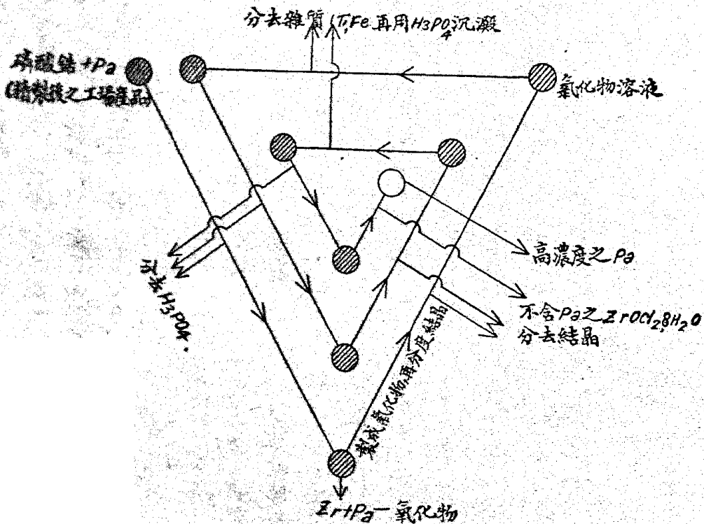
第二圖 螺旋製濃手續
