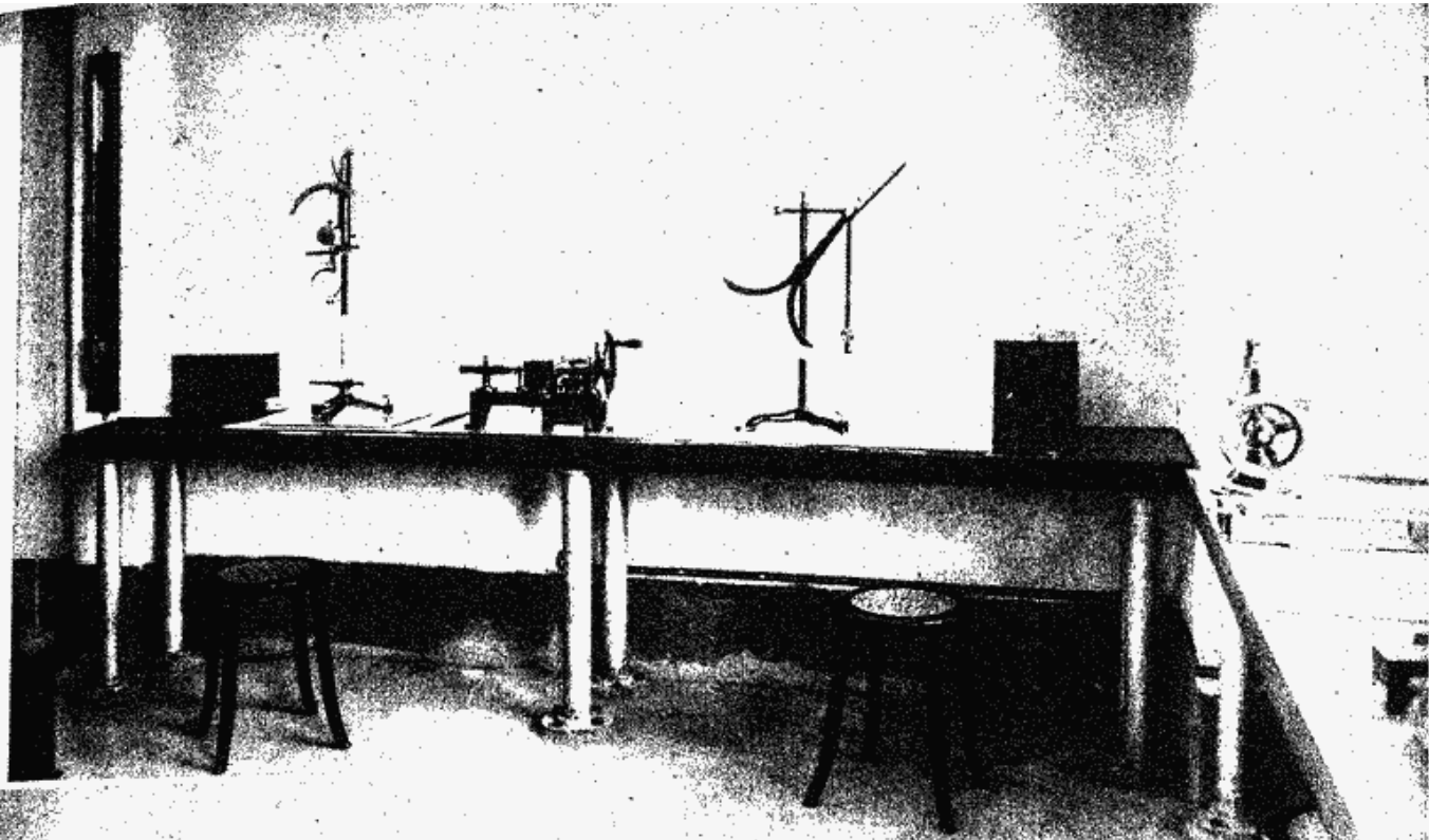
→ 試驗紙張儀器之一
