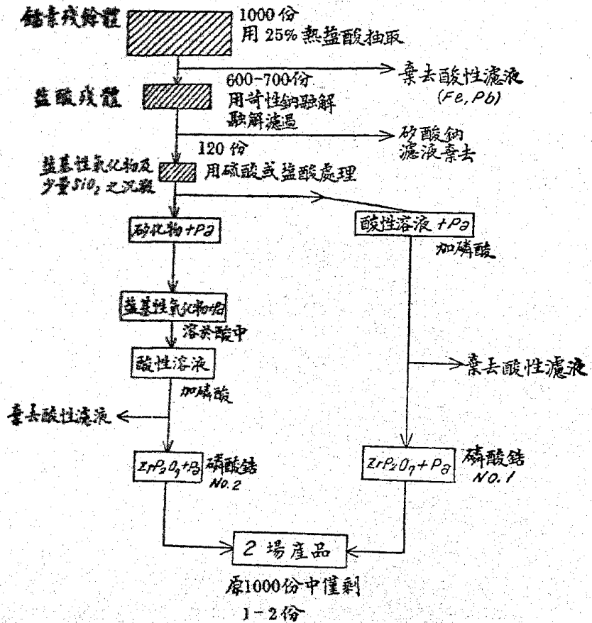
第一圖 鈷素提取之工業手續
