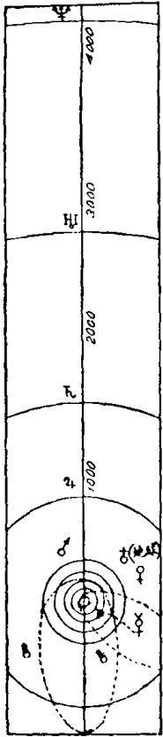
第二圖 太陽系
