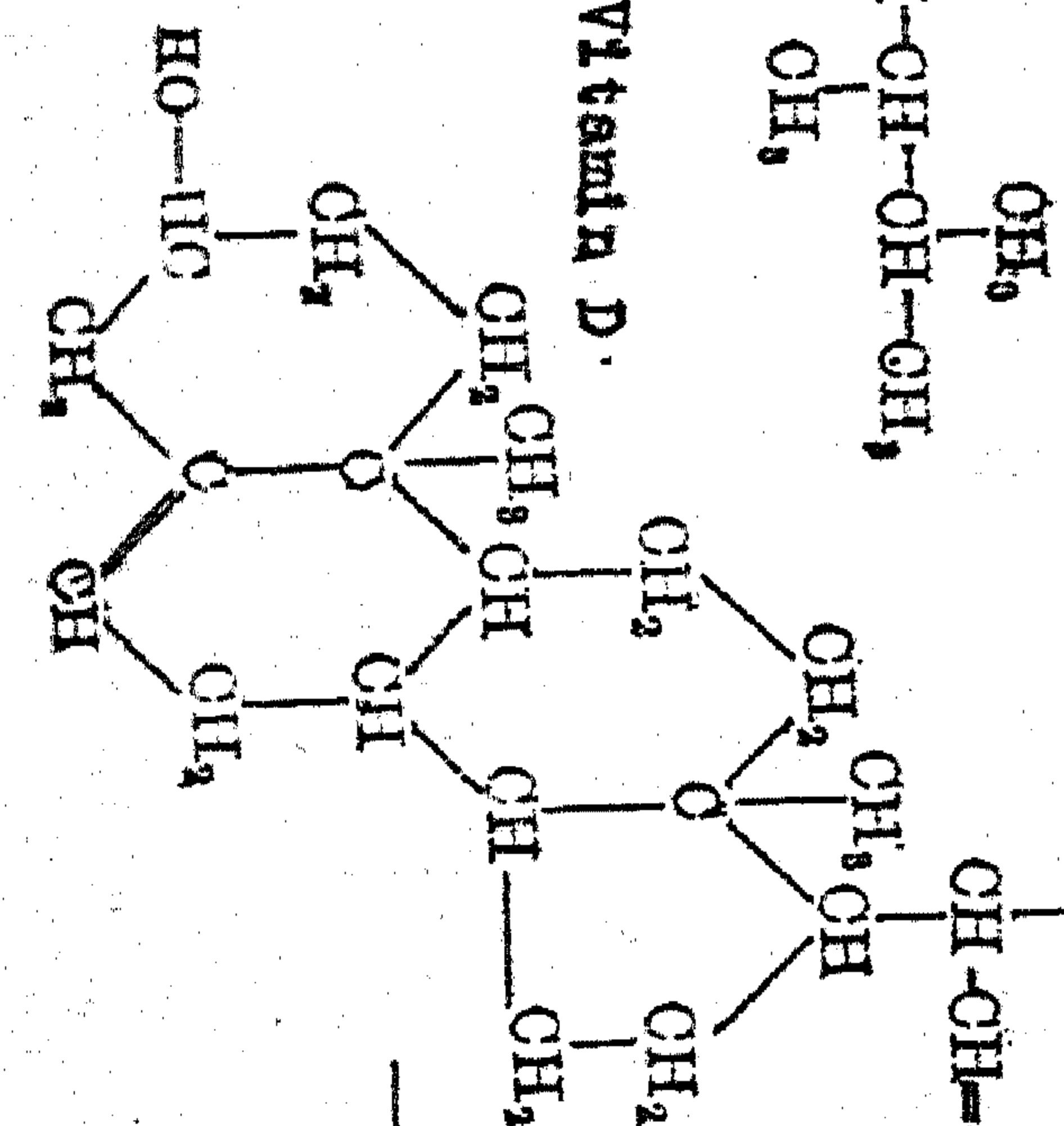
XI. Stigmasterin
