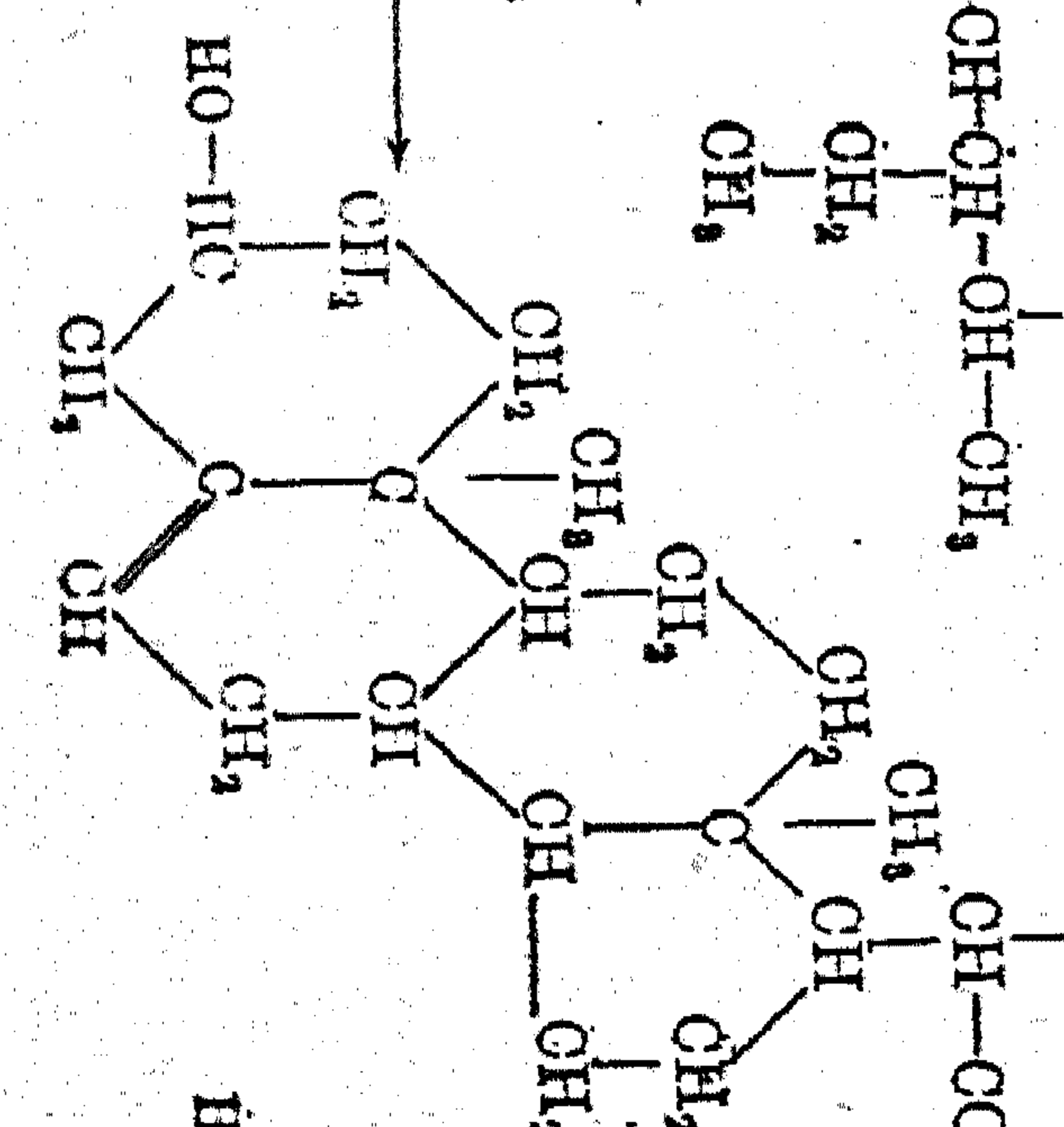
XII.
