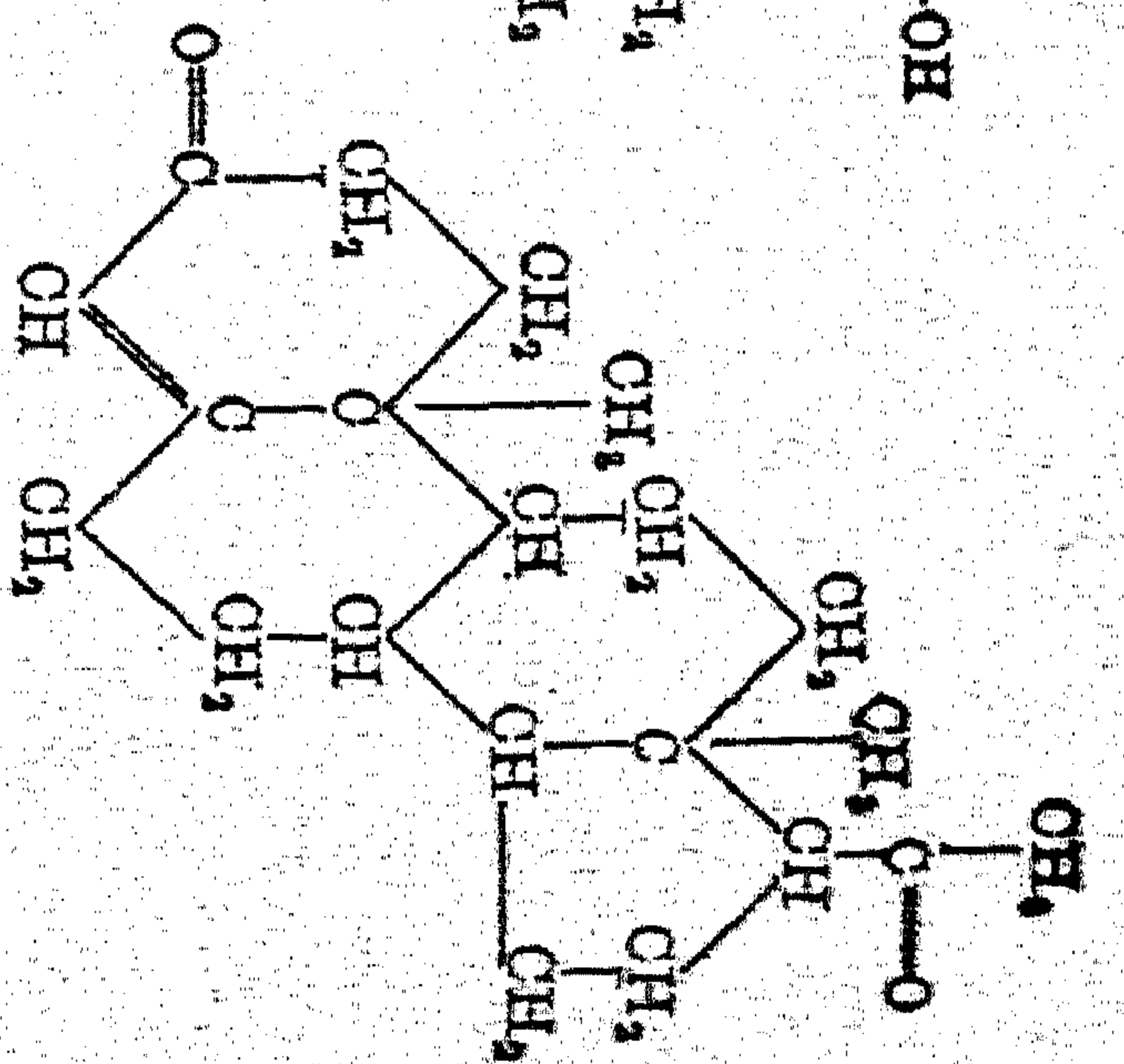
V. Corpus-luteum-Hormon
