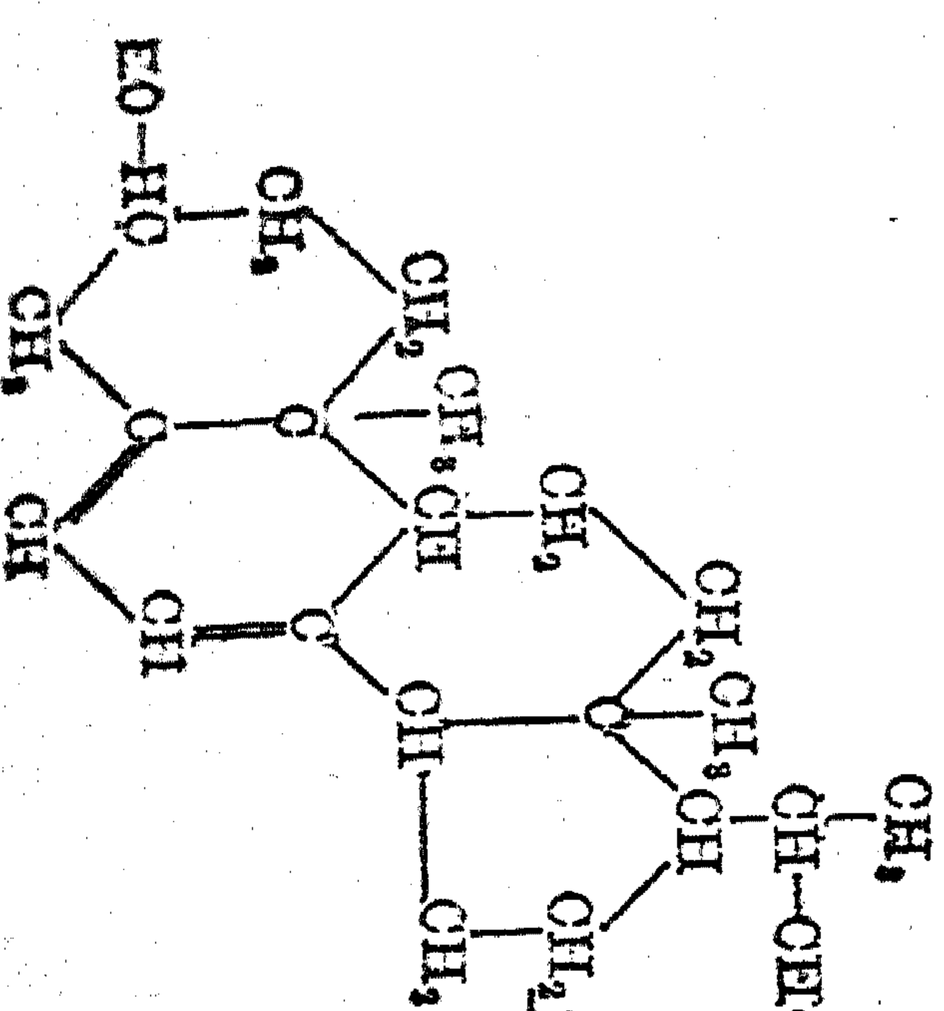
Vitamin D.
