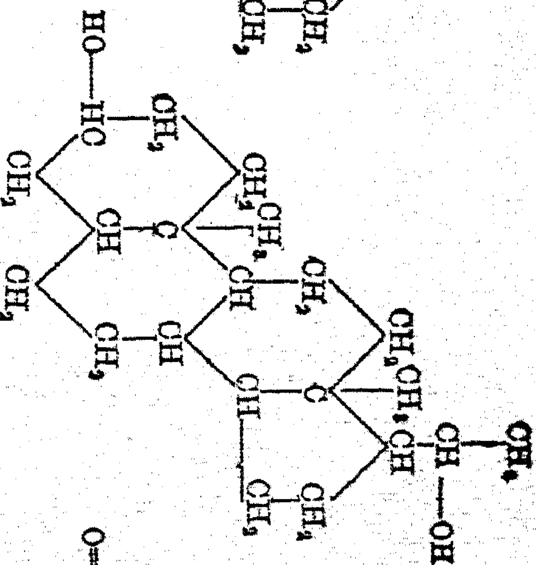
IV. Pregnandiol
