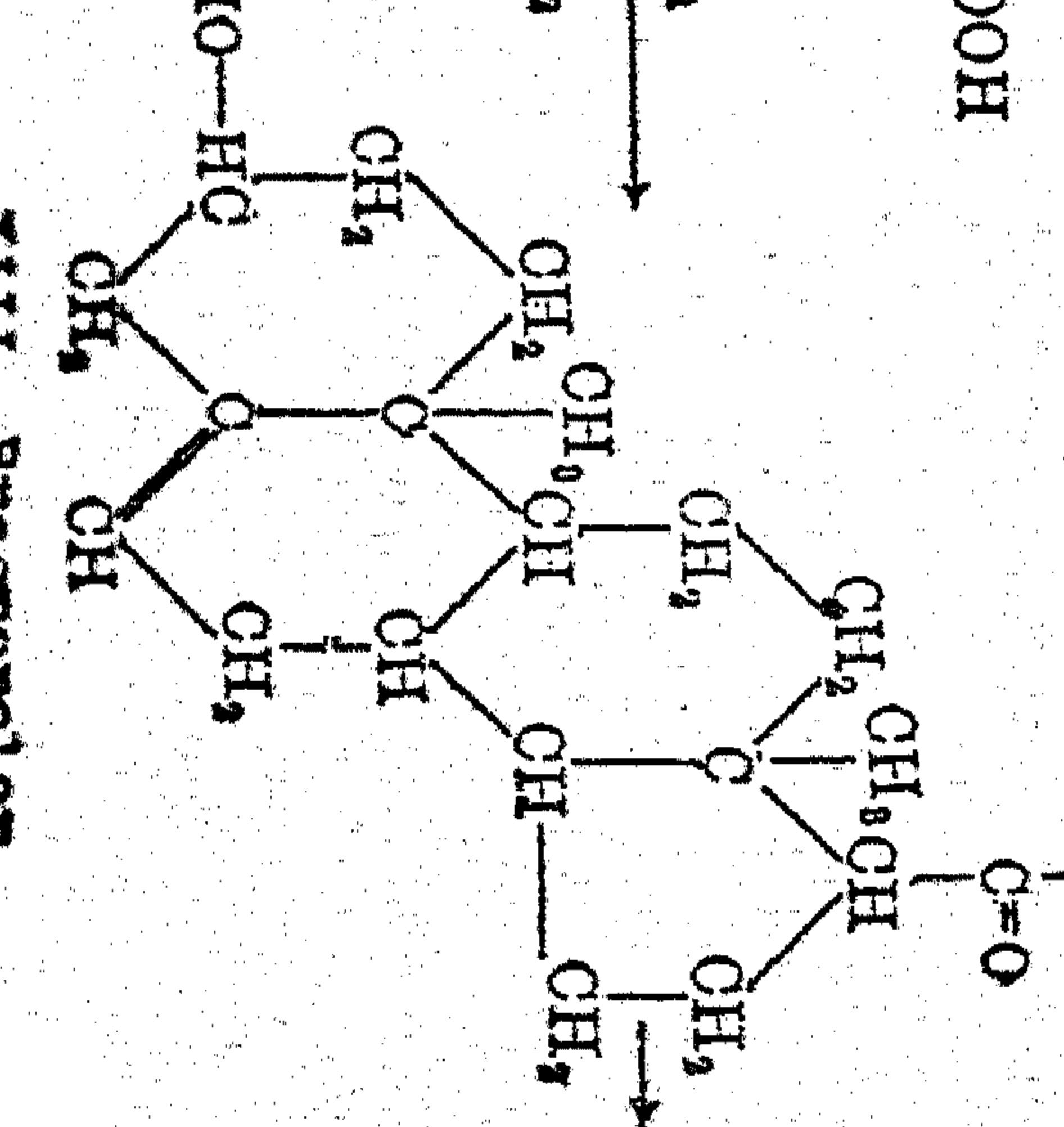
Corpus-luteum-Hormon
