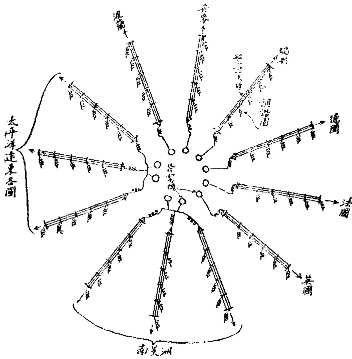
紐約無線電總站天線組系統之全圖
