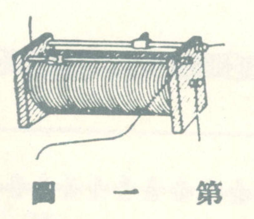
旋轉誘導調音圈 Vari Coupler (四) 蛛網或線圈 Spiderweb Coil (五) 竹籃式線圈 Low Loss Vari Coupler
