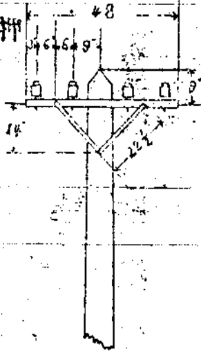
(四綫木担一條時)
