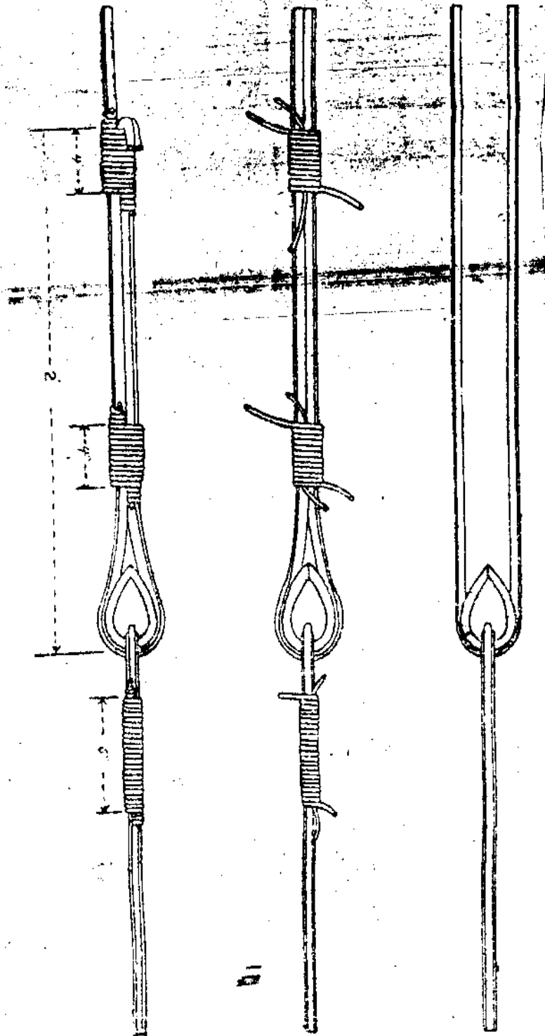
環緊接續圖
