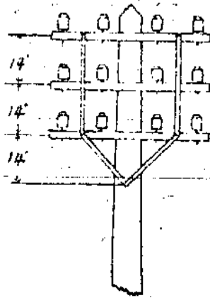
押條及撐脚裝置圖
