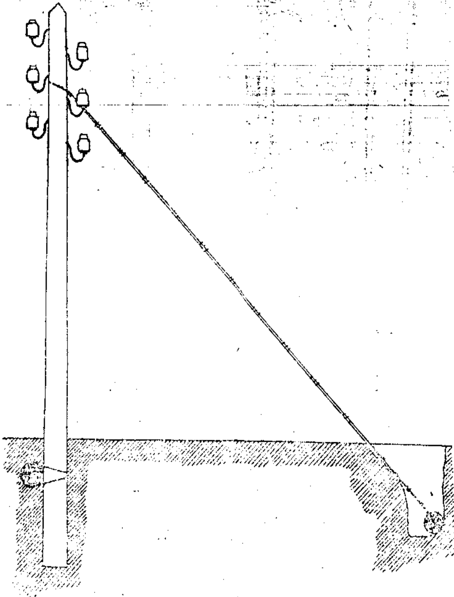
拉綫圖
