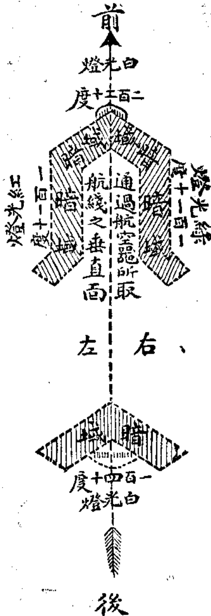
航空器信燈圖式
