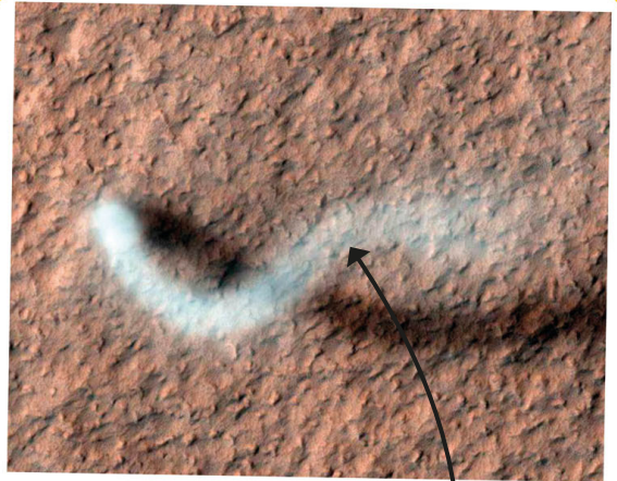
Dust devil
